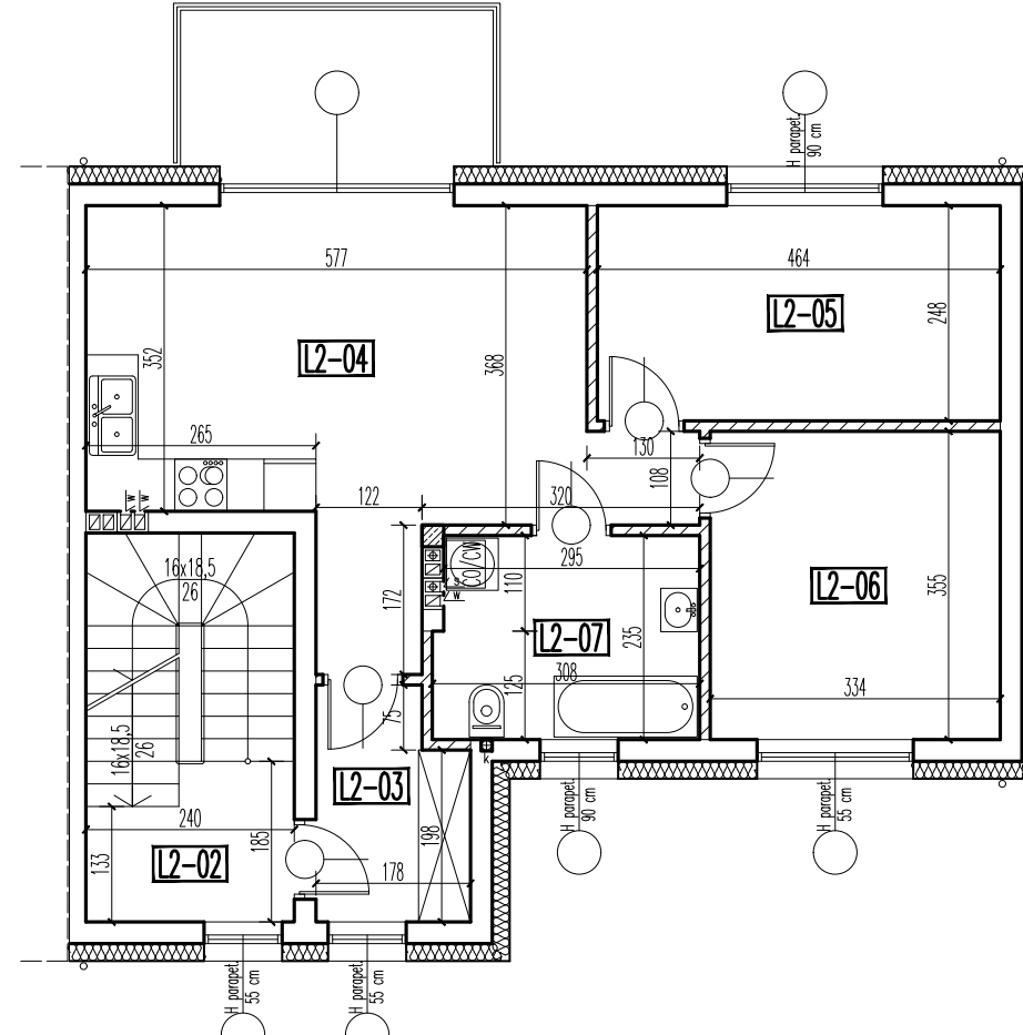
RZUT PIĘTRA
