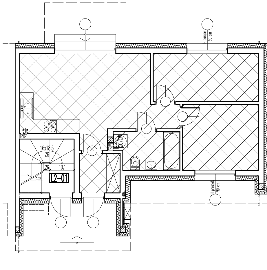
RZUT PARTERU
